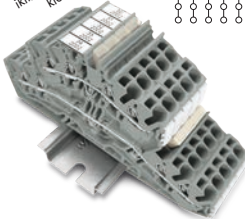
ikili sonsuz köprü sistemi istediğiniz kadar klemensli köprülemek için tek tip
