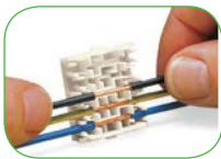
İzolesi açılmış iletkeni kablo yuvasına yerleştirin. Yuva standart soket yerine kullanılır.
