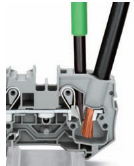
Sadece bakır, yüksük yok, gevşeme saçaklanma ve ark yok!
