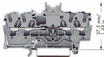
Bir gövdede iki klemens. Her iki tarafta etiketlenebilir, 2 katlı klemens yerine kullanılır
